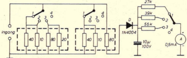
Fig. 1. Schakeling van de wattmeter: Schakelaarposities: 1 :: 4 \Omega , 2 :: 8 \Omega , 3 :: 16 \Omega , 4 :: uit. De stippe lijntjes omsluiten telkens een combinatieweerstand.
